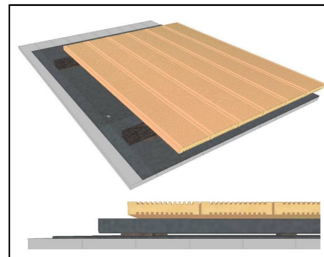
03.1.7 Lattenrost aus sib. Lärche auf Abdichtung 28/146 auf Lücke gesetzt mit Kunststoff-Unterprofil auf Gummipads
