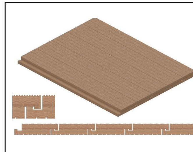
03.1.2 wasserführender Holzfußboden aus sib. Lärche mit Rieselschutz 45 x 145 mm HTL-Kehlbodensystem
