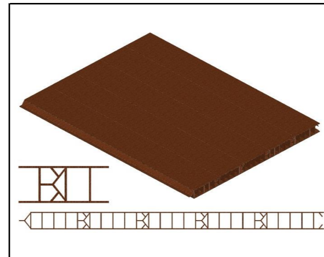
03.1.3 Werzalit Terraza-Boden-System Nut-Feder-System wasserdicht verlegt 38 x 145 mm
