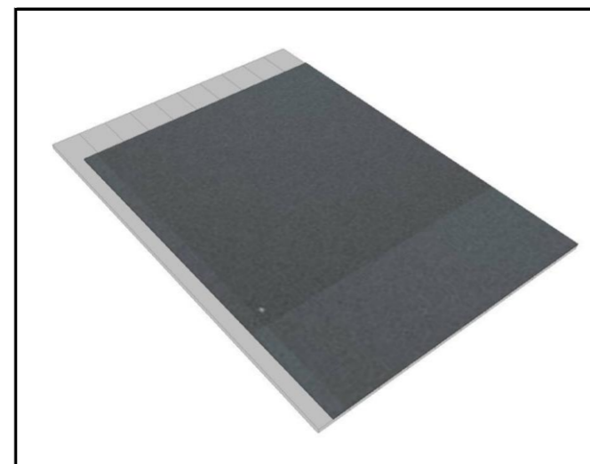
03.1.6 Systemabdichtung auf Holzschalung Bitumen-Kaltselbstklebebahn Polyesterverbundträgerinlage durchwurzelungssicher Flachdach mit Dachneigung 2%....7% EPDM-System fugenlos durchwurzelungssicher 0°....20°
