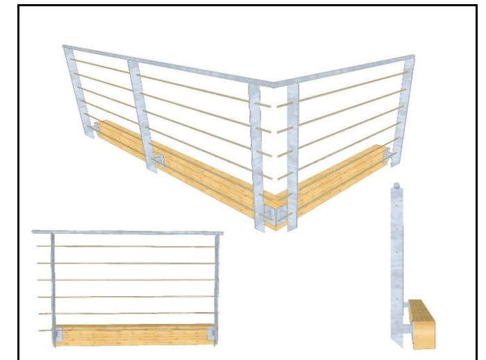
GST 8 Geländer aus Stahl, verzinkt Montage an Träger seitlich angesetzt Stützen aus Flachmaterial waagerechte Edelstahlstangen 10 mm Lücke 120 mm Handlauf Edelstahl rund 42 mm
