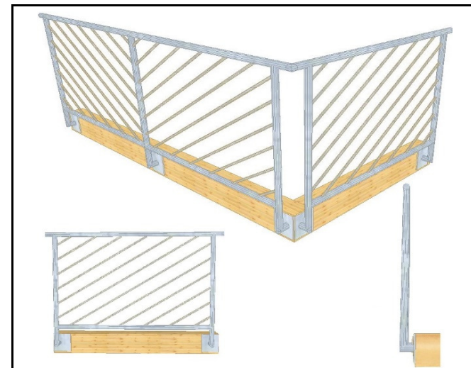
GST 4 Geländer aus Stahl, verzinkt Montage an Träger seitlich angesetzt Ober- und Untergurt rund 42 mm diagonale Stäbe rund 16 mm Lücke 120 mm
