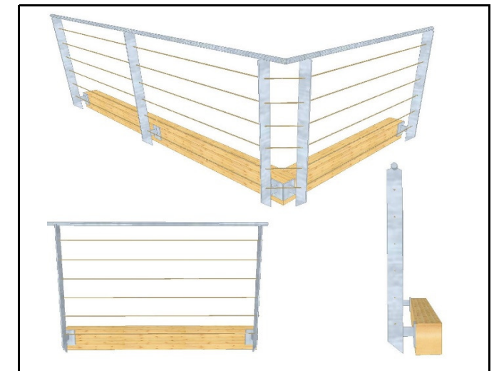
GST 7 Geländer aus Stahl, verzinkt Montage an Träger seitlich angesetzt Stützen aus Flachmaterial waagerechte Edelstahlseile 5 mm Lücke 120 mm Handlauf Edelstahl rund 42 mm
