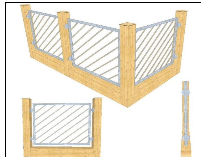
GST 3 Geländer aus Stahl, verzinkt Montage zwischen Stützen Ober- und Untergurt rund 42 mm diagonale Stäbe rund 16 mm Lücke 120 mm
