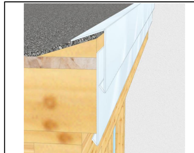
09.1. HTL®-Rand-Balkenabdeckung aus Alu 3.3 für Systemabdichtung mit Aufdachdämmung
