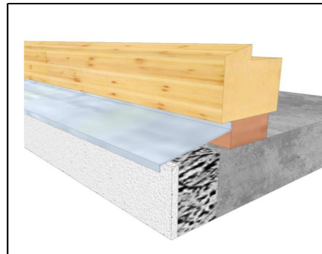
09.1.7 Sockelverblechung aus Aluminium Wintergarten
