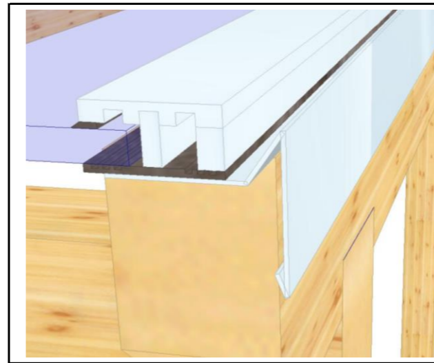
09.1.3 HTL®-Rand-Balkenabdeckung aus Alu für Doppelstegplatte/Glas
