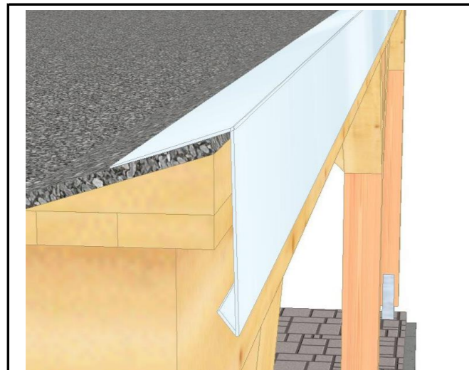
09.1. HTL®-Rand-Balkenabdeckung aus Alu 3.2 für Systemabdichtung
