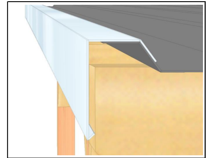
09.1. HTL®-Rand-Balkenabdeckung aus Alu 3.1 für Trapezblech
